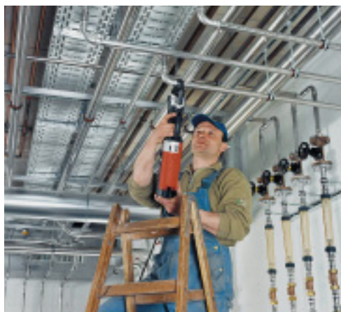
Insgesamt 12.900 lfm Edelstahlrohre (DN 15-150, Werkstoff-Nr. 1.4401) wurden in der Unfall- klinik Murnau verbaut.
